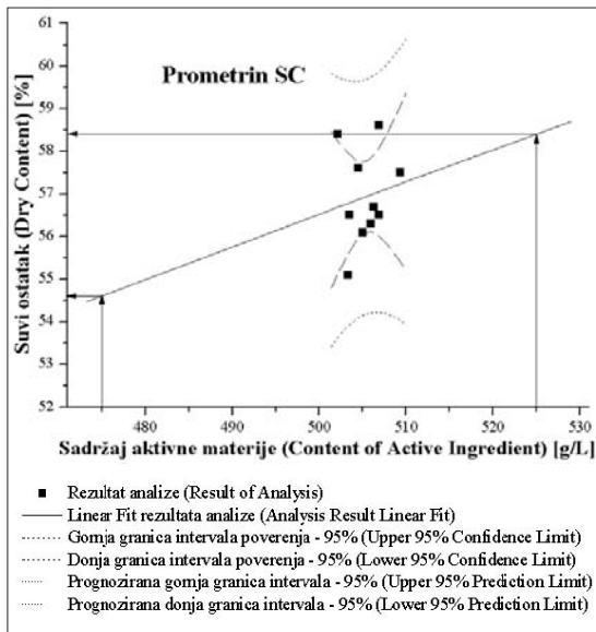
Slika 2. Funkcionalna zavisnost sadržaja suvog ostatka i sadržaja aktivne materije za preparat Prometrin SC Figure 2. Relation between dry content and content of active ingredient for formulation Prometrin SC
