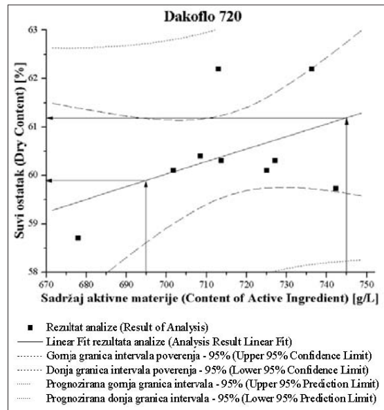
Slika 4. Funkcionalna zavisnost sadržaja suvog ostatka i sadržaja aktivne materije za preparat Dakoflo 720 Figure 4. Relation between dry content and content of active ingredient for formulation Dakoflo 720
