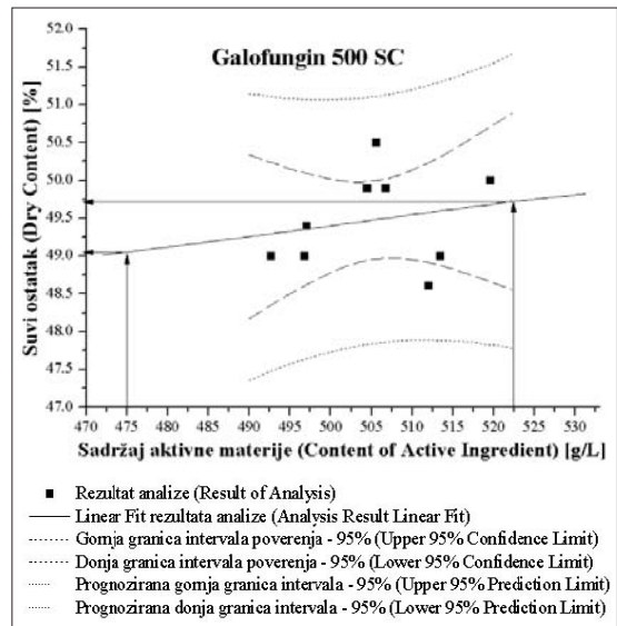
Slika 5. Funkcionalna zavisnost sadržaja suvog ostatka i sadržaja aktivne materije za preparat Galofungin 500 SC Figure 5. Relation between dry content and content of active ingredient for formulation Galofungin 500 SC
