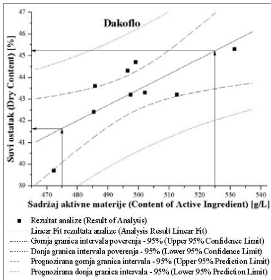
Slika 3. Funkcionalna zavisnost sadržaja suvog ostatka i sadržaja aktivne materije za preparat Dakoflo Figure 3. Relation between dry content and content of active ingredient for formulation Dakoflo
